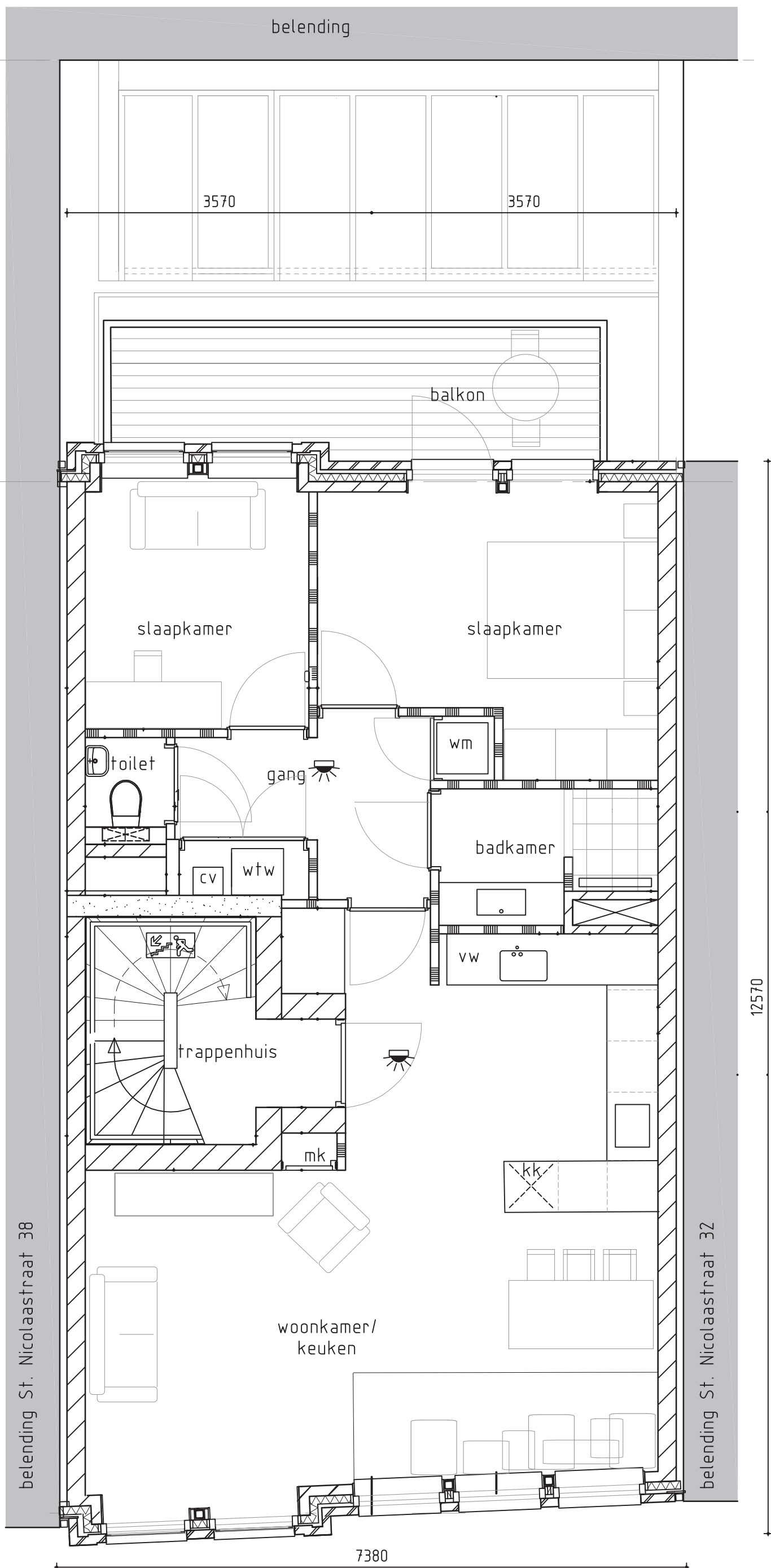
1e VERDIEPING
